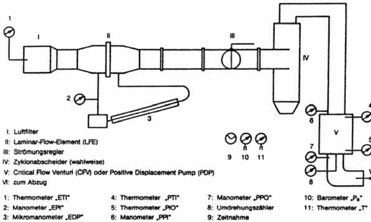
Abbildung 2: Schematische Darstellung einer Kalibriervorrichtung für CVS-Geräte
