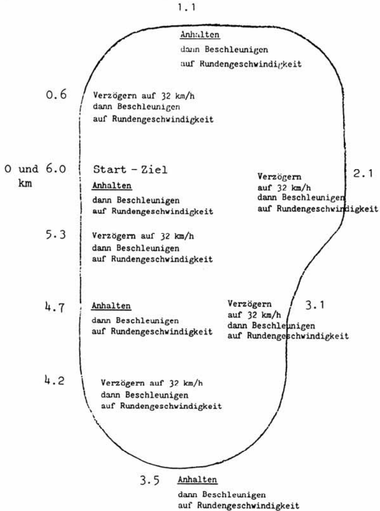
Abbildung 1: Programm für den Fahrbetrieb
