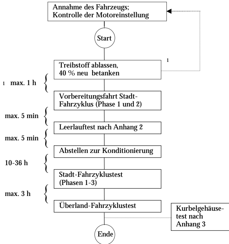
Abbildung 2: Fremdzündungsmotoren / Prüfablauf wenn nur Abgasemissions-Messungen
