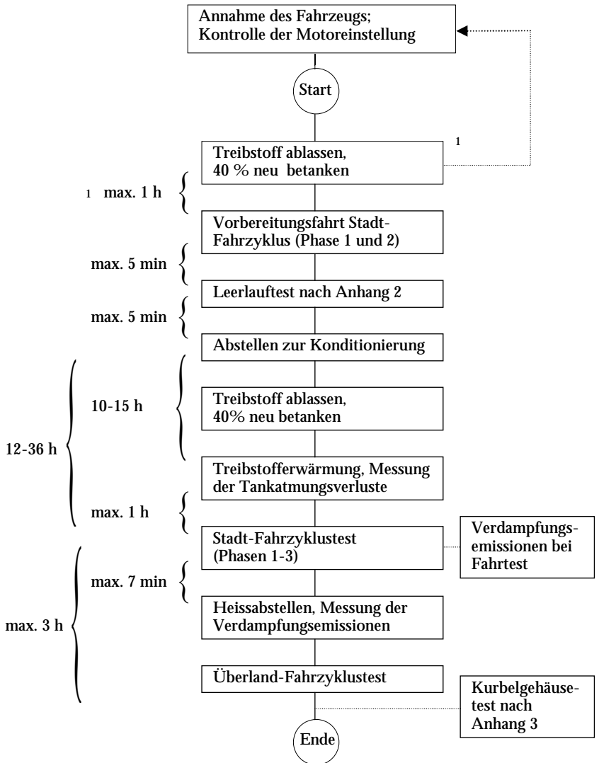
Abbildung 1: Fremdzündungsmotoren / Prüfablauf für die Abgas- und Verdampfungsemissions-Messungen
