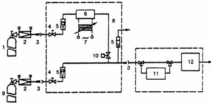
Abbildung 1: Schaltschema für \text{NO}_2 - \text{NO} -Konverterprüfung
